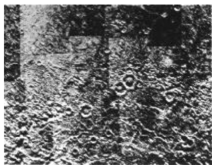
Cuenca CALORIS PLANITIA
