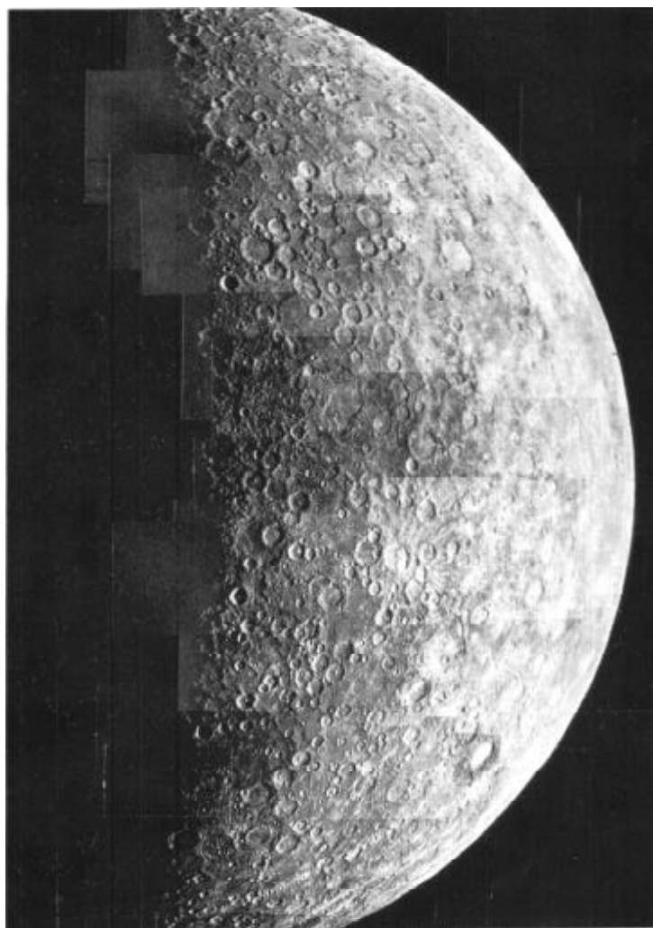
composición fotográfica de Mercurio, obtenida elaborando las imágenes captadas por la sonda Mariner 10 en marzo de 1974.
